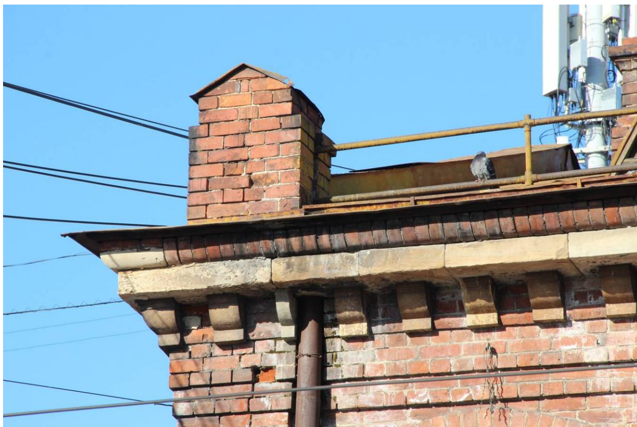
Видовая точка № 4. Фрагмент венчающего карниза главного фасада (Верховая К.Е., 09.04.2021 г.)
