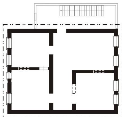
План 2 этажа
