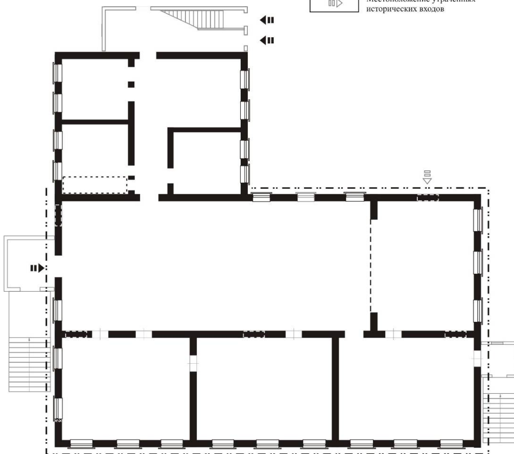
План 1 этажа
